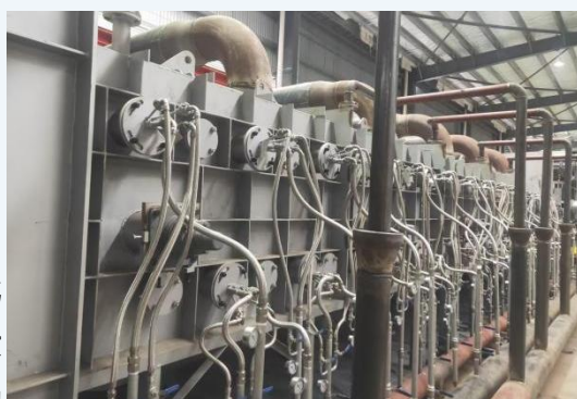
湖南宏旺常化 酸洗线气雾喷 淋安装现场
