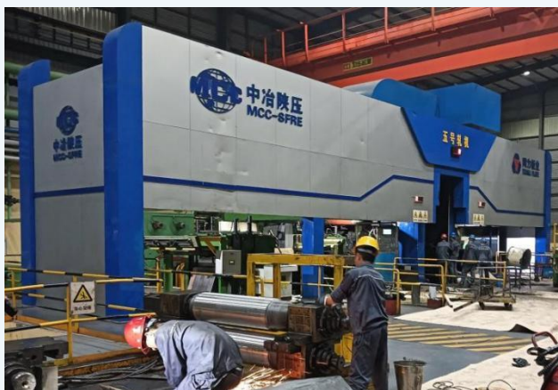
单机六辊轧机现场 (1)
