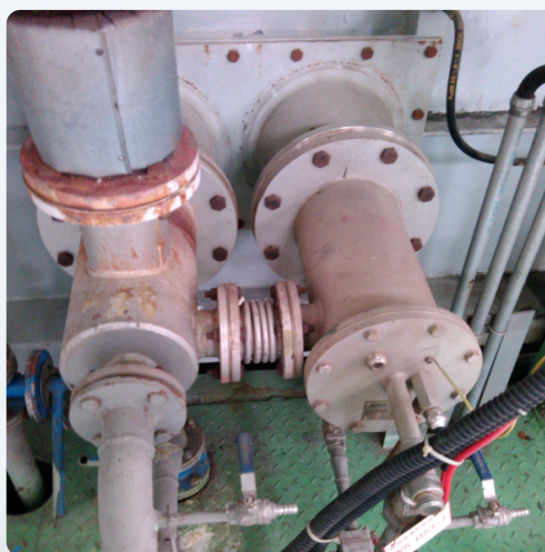
● 辐射管烧嘴在武钢现场
